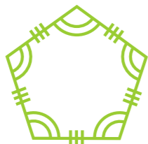
Pięciokąt foremny
