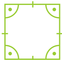
Kwadrat
