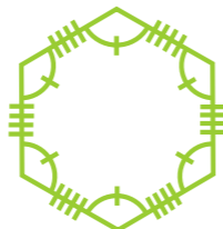
Sześciokąt foremny
