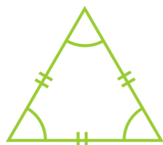
Trójkąt równoboczny
