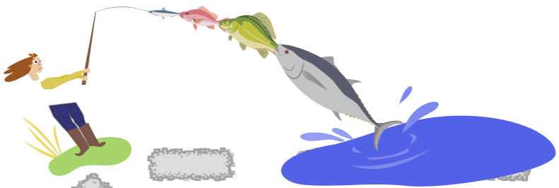
ciąg rosnący
